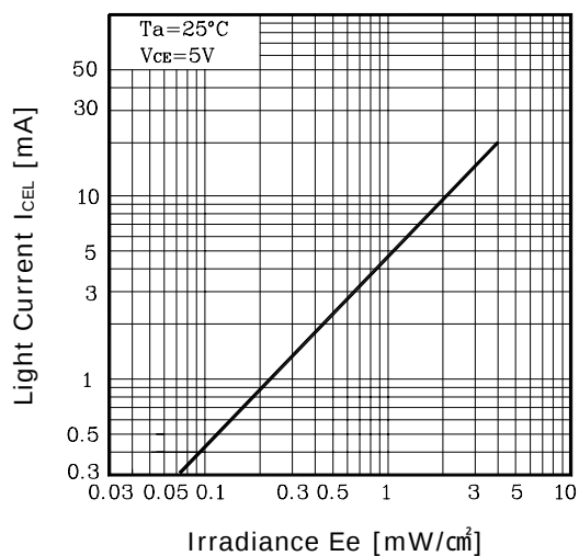
Fig. 1 I_{CEL} - E_e
