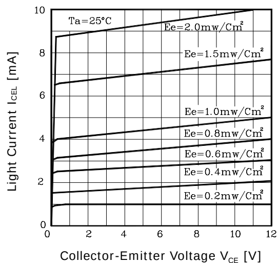
Fig. 2 I_{CEL} - V_{CE}
