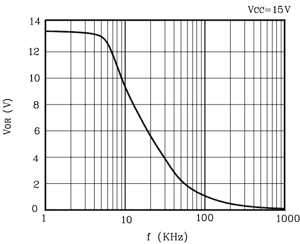
Fig. 6 V_{OR} -f
