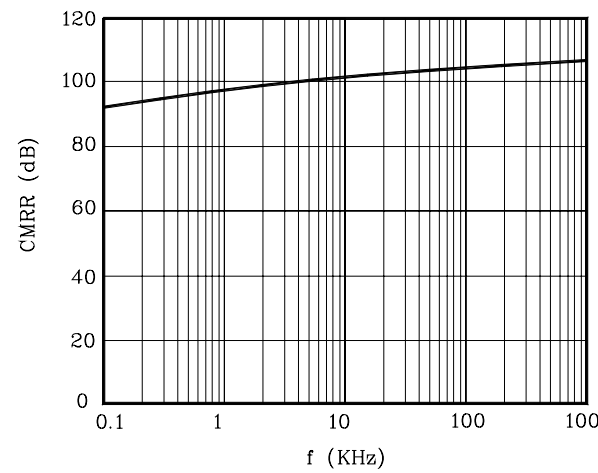
Fig. 5 CMRR-f
