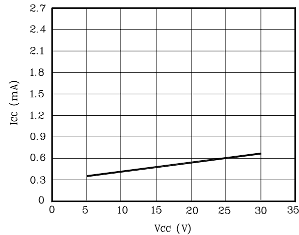
Fig. 1 I_{CC} - V_{CC}
