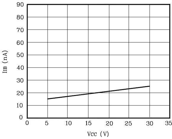
Fig. 2 I_{IB} - V_{CC}
