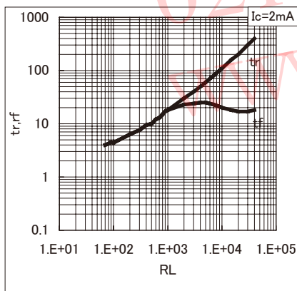
■応答時間/負荷抵抗特性 *1 t_r, t_f(\mu\text{sec})/R_L(\Omega)
