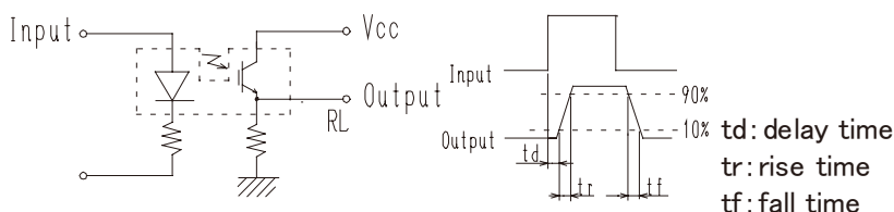
*1 応答時間特性図
