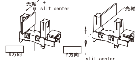
*2 位置検出特性図
