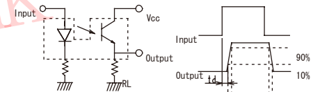
*1応答時間特性図
