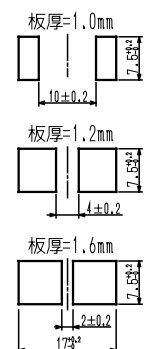
推奨取付寸法
