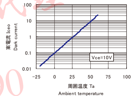
■暗電流/周囲温度特性 I_{ceo}(\text{nA})/T_a(^{\circ}\text{C})
