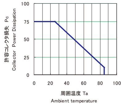
■コレクタ損失/周囲温度 P_c(\text{mW})/T_a(^{\circ}\text{C})
