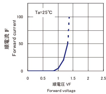
■順電流/順電圧特性 I_F(\text{mA})/V_F(\text{V})
