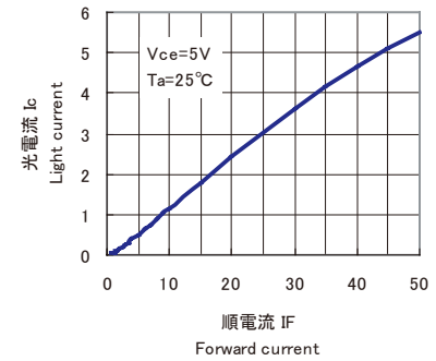
■光電流/順電流特性 I_c(\text{mA})/I_F(\text{mA})
