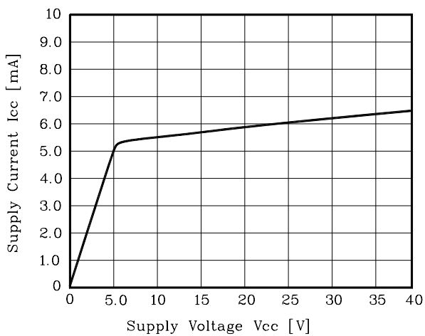
Fig. 5 I_{CC} - V_{CC}
