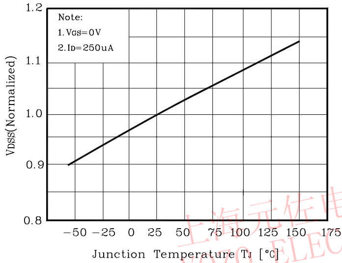
Fig. 7 V_{DS} - T_J
