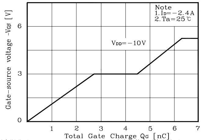
Fig. 6 V_{GS} - Q_G
