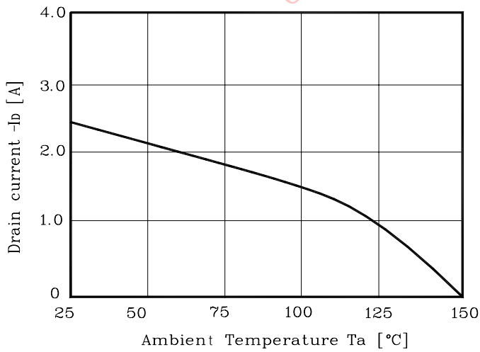
Fig. 9 I_D - T_a
