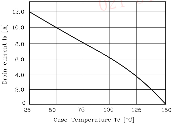
Fig. 9 I_D - T_C
