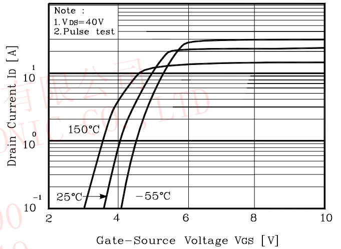
Fig. 2 I_D - V_{GS}
