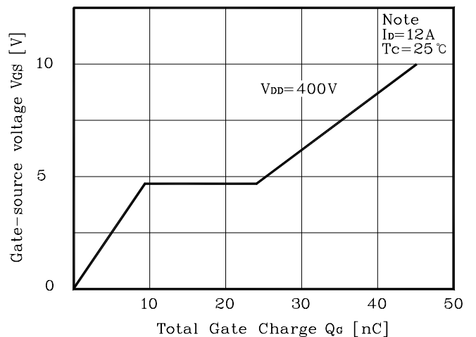
Fig. 6 V_{GS} - Q_G
