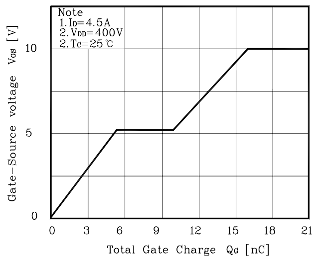
Fig. 6 V_{GS} - Q_G
