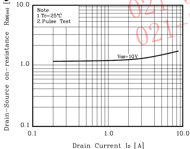
Fig. 3 R_{DS(on)} - I_D
