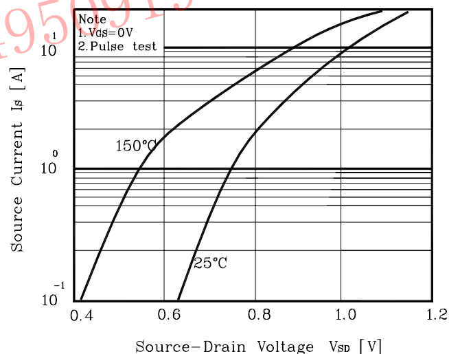
Fig. 4 I_S - V_{SD}
