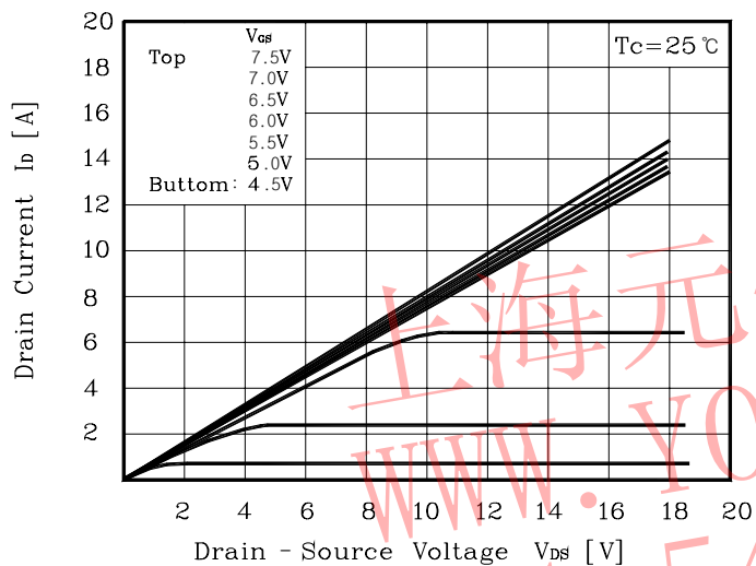
Fig. 1 I_D - V_{DS}
