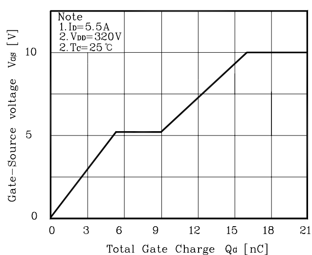
Fig. 6 V_{GS} - Q_G
