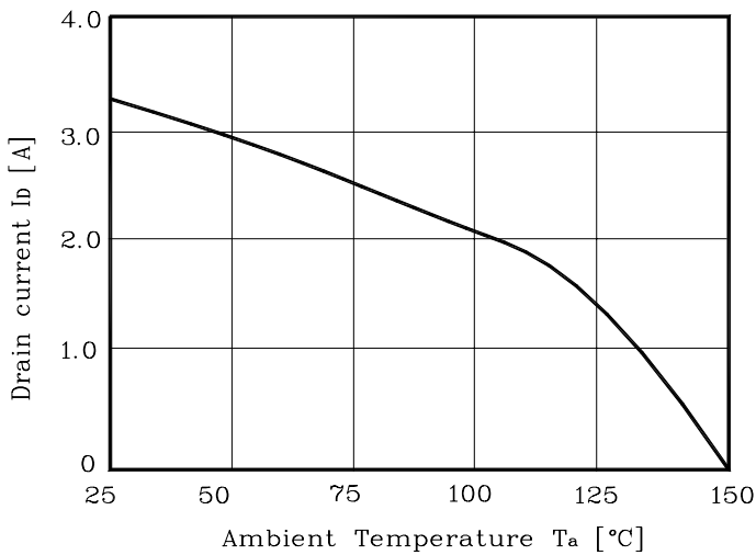
Fig. 9 I_D - T_a
