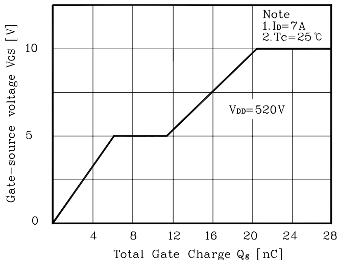
Fig. 6 V_{GS} - Q_G
