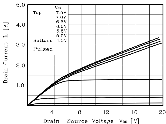
Fig. 1 I_D - V_{DS}
