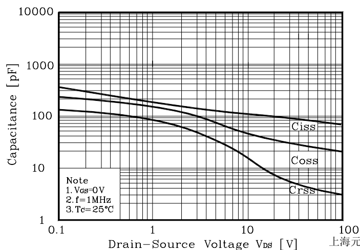
Fig. 5 Capacitance - V_{DS}
