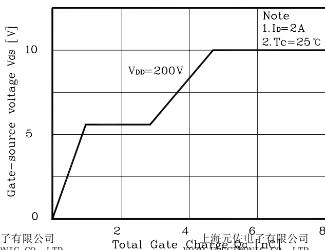
Fig. 6 V_{GS} - Q_G
