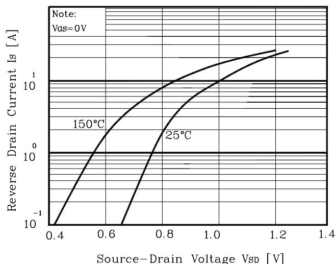
Fig. 4 I_S - V_{SD}
