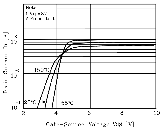
Fig. 2 I_D - V_{GS}
